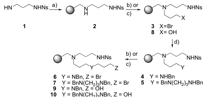
Scheme 1. (a) Merrifield resin, DIEA, 50 °C. (b) 1,3-Dibromopropane, DIEA, 50 °C. (c) 3-Bromopropanol, DIEA, 50 °C. (d) Benzylamine or N,N' -dibenzylpropane-1,3-diamine, DIEA, 50 °C.
